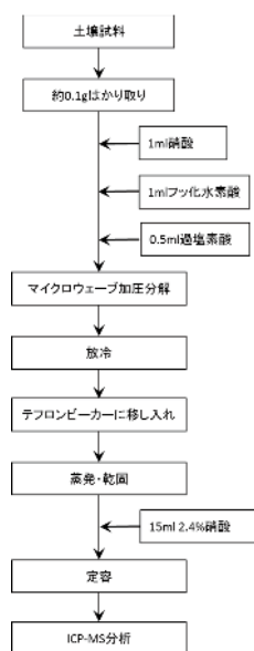
図 4 土壌中の重金属の分析手順
