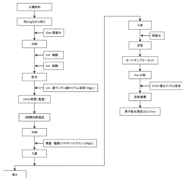
図 2 土壌中の総水銀の分析手順
