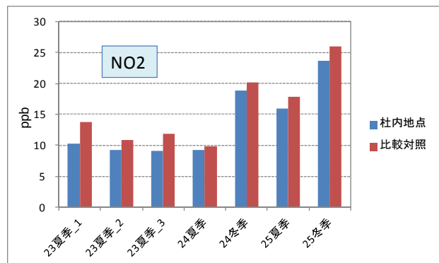
図11 杜内平均濃度と比較対照濃度（NO 2 ）
