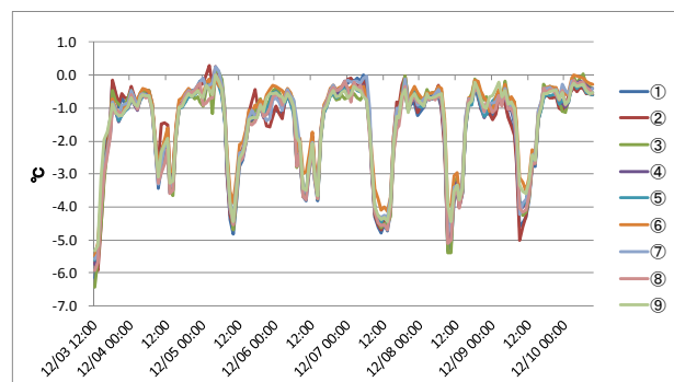
図 9 温度差の経時変化（2012/12/3-10）
