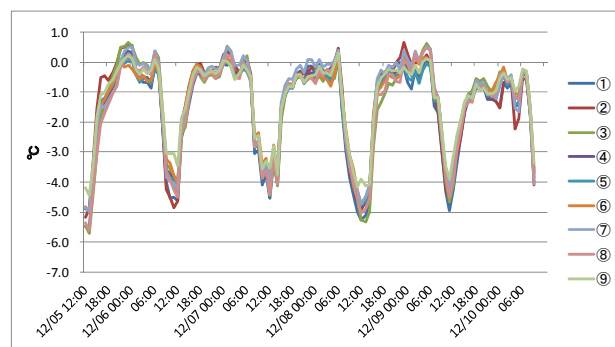
図 10 温度差の経時変化（2013/12/5-10）
