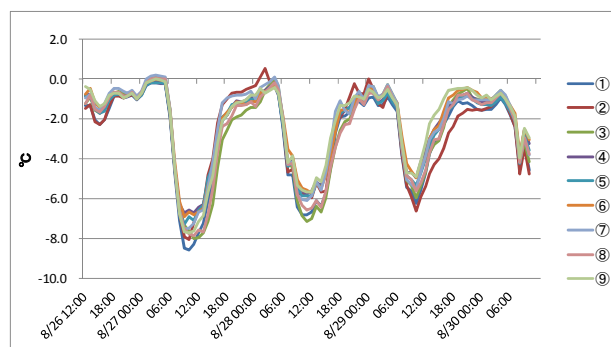
図8 比較対照との温度差の経時変化(2013/8/26-30)
