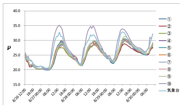
図7 温度の経時変化(2013/8/26-30)
