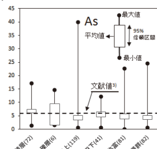
図 2 各地層中の砒素濃度
