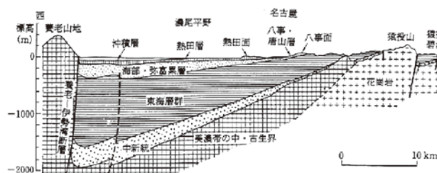
図 1 濃尾平野の地下断面図 2)
