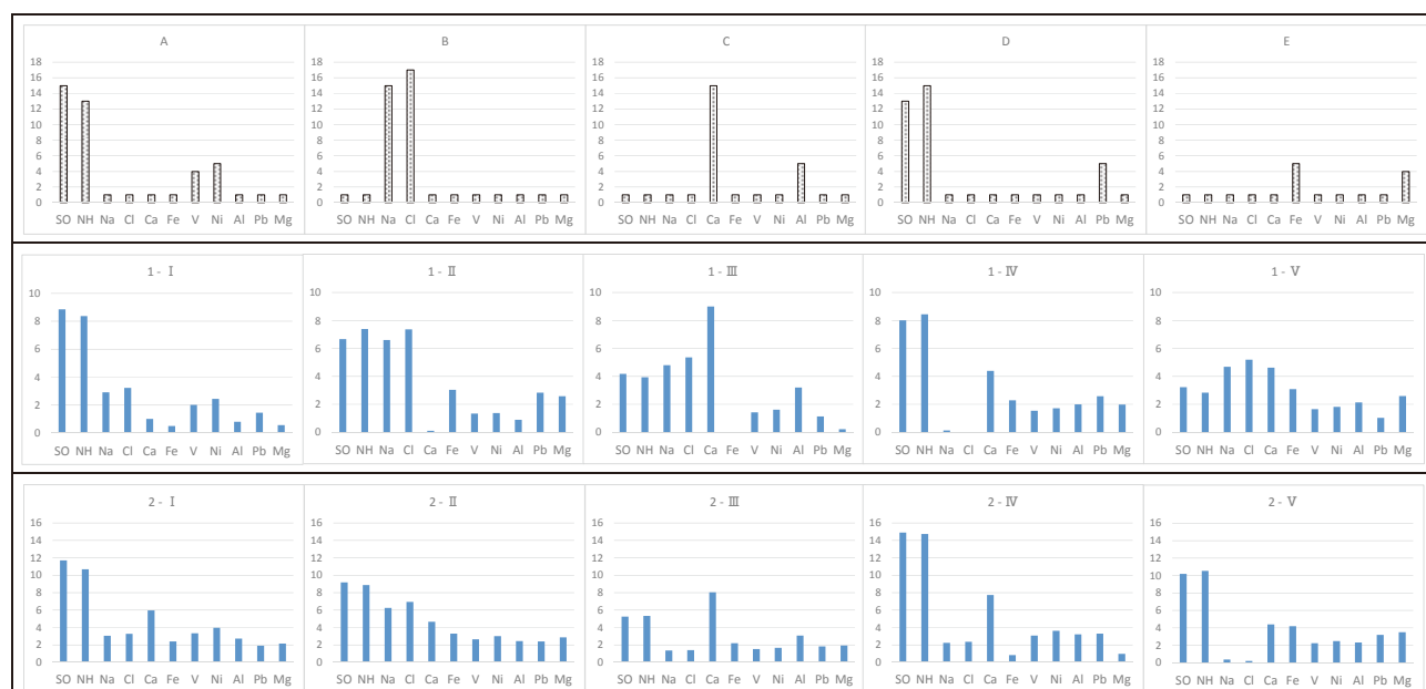
Fig.1 仮定した発生源データ（上段）および PMF 結果（case1：中段，case2：下段）
