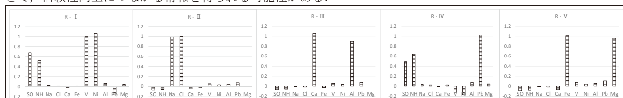
Fig.2 関数 fa()による因子分析結果[case1]
