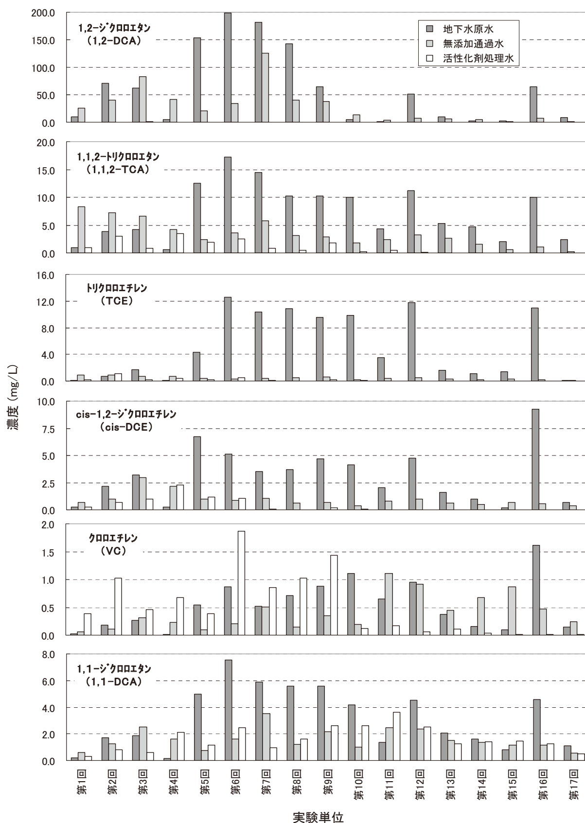
図6 活性化剤による脱塩素化の促進
