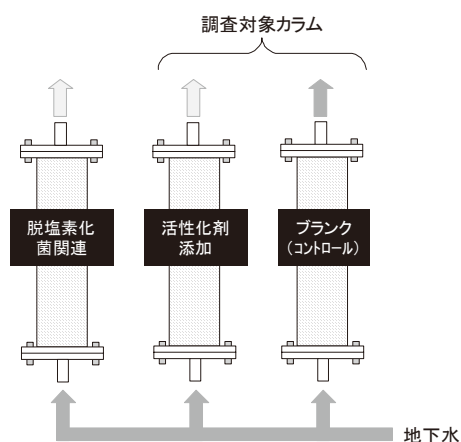
図 2 砂充填カラム実験装置の概略
