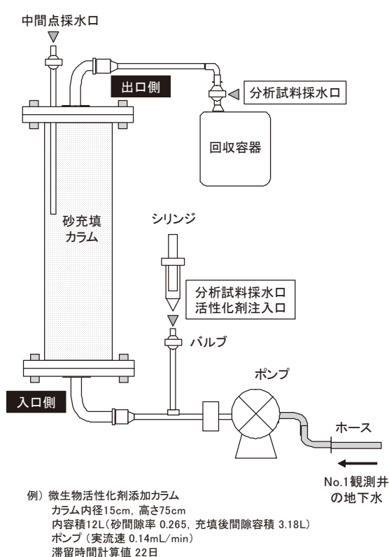
図 2 砂充填カラム実験装置の概略
