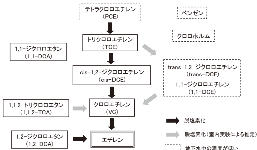
図3 脱塩素化反応によるVOCの嫌気分解
