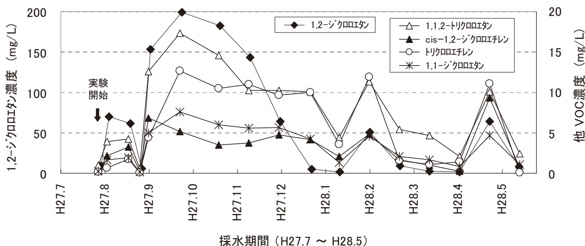
図 5 地下水原水の VOC 濃度の変化
