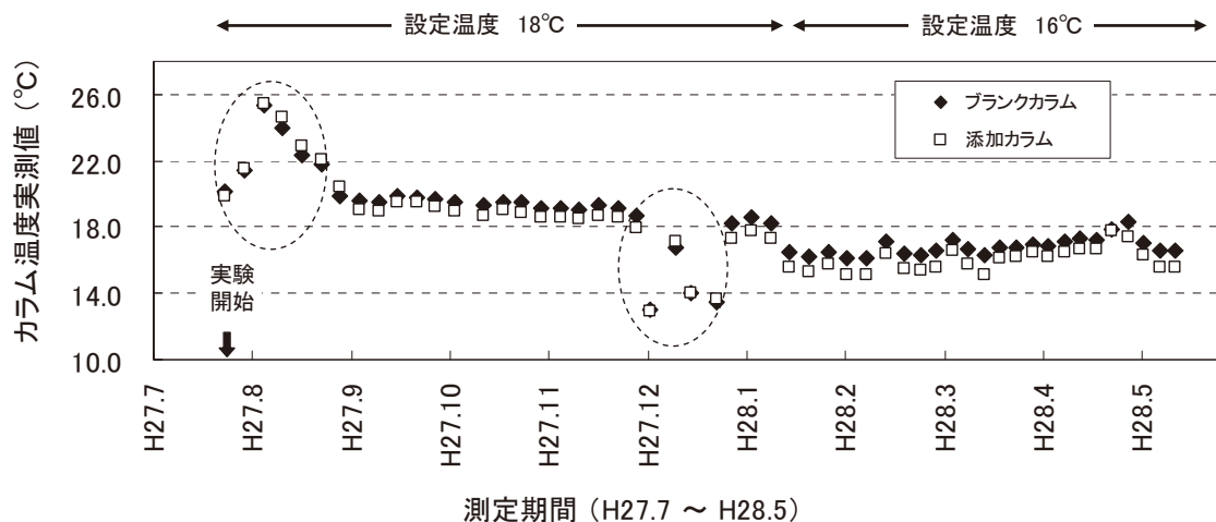
図 4 実験カラムの温度変化
