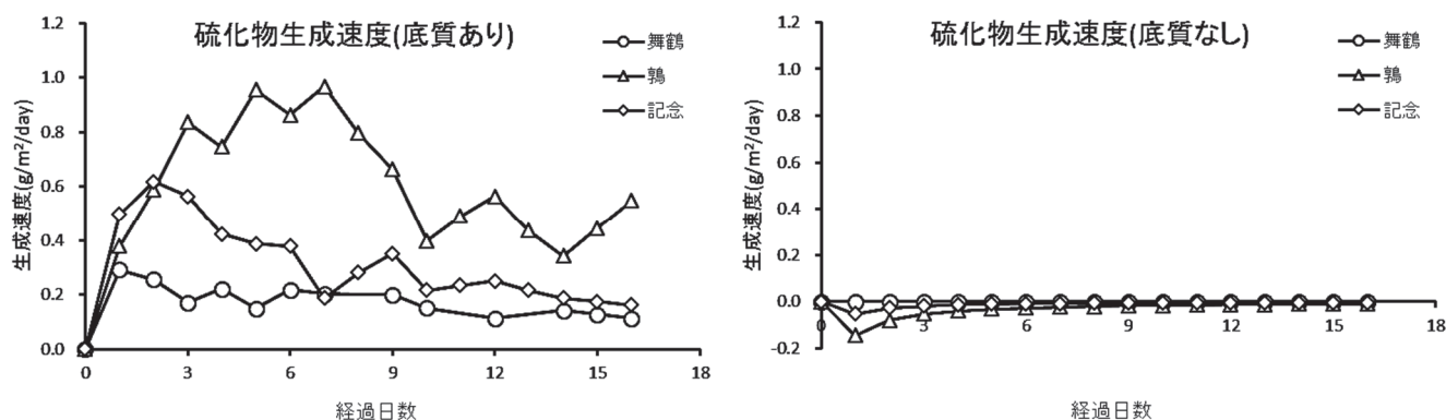
図 5 各地点の硫化物生成速度
