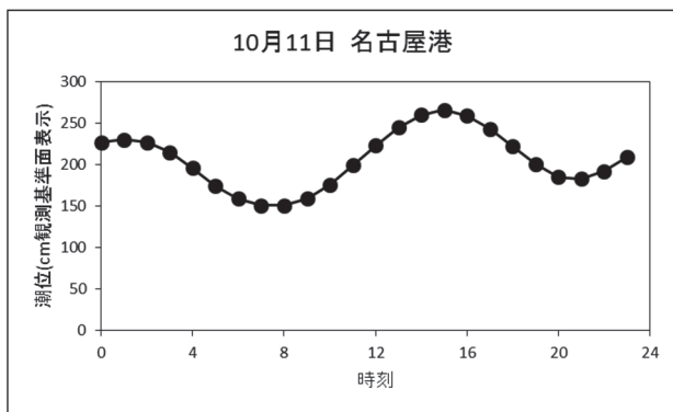
図2 調査日の潮位変動
