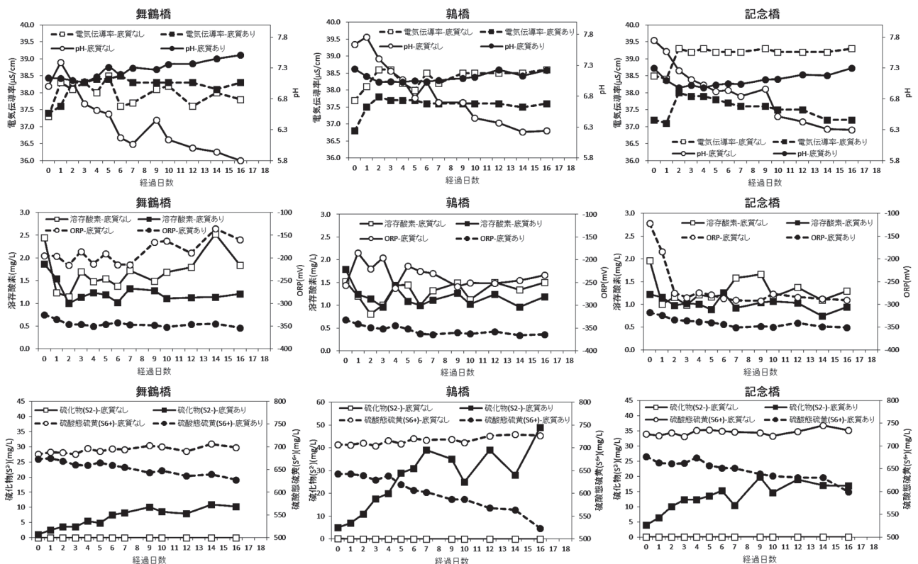
図4 室内カラム実験の経日測定結果
