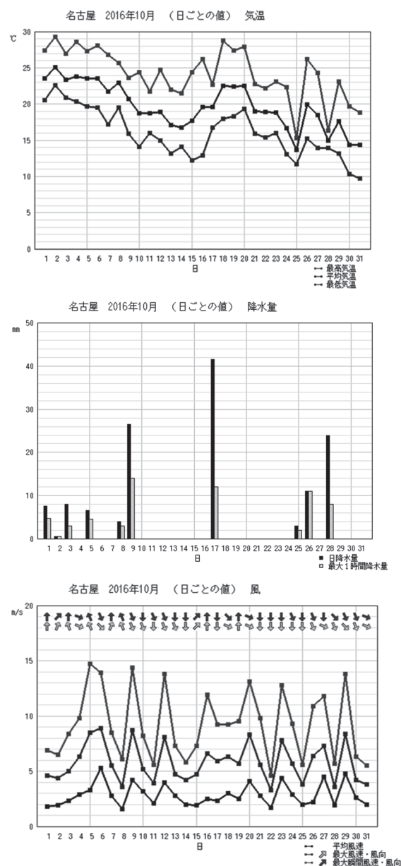
図1 調査月の気象データ
