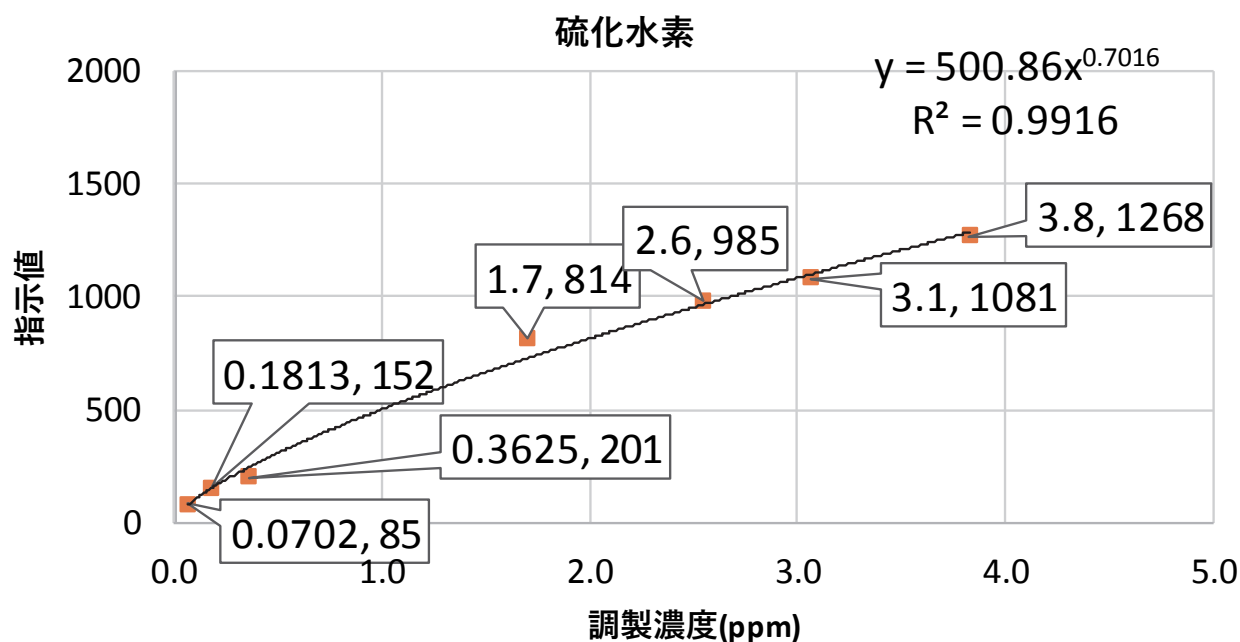
図 2 硫化水素測定結果
