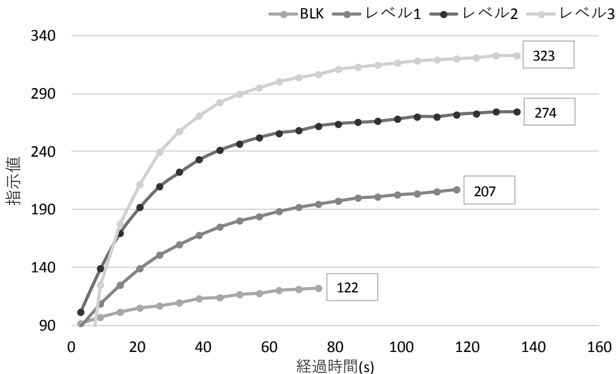
図1 硫化水素濃度別ニオイセンサ指示値
