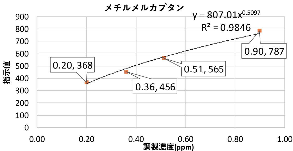
図 3 メチルメルカプタン測定結果
