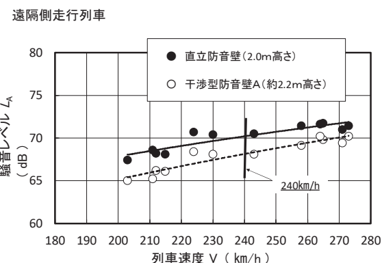
図 7 直立防音壁と干渉型防音壁 A の比較 (騒音レベルと列車速度の関係)
