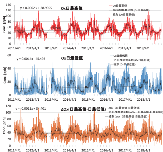
図3 O 3 濃度日最高値（上段）、日最低値（中段）、ΔO 3 （日最高値-日最低値）（下段）の経年変化（惟信高校）
