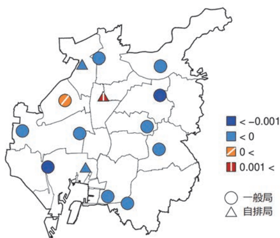
図4 ΔO 3 （日最高値-日最低値）の経年変化（2011～2018年度）の回帰直線の傾き
