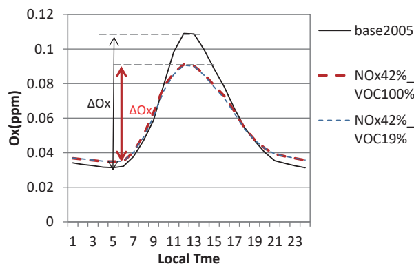
図 2 シミュレーションモデルにより計算した Ox 濃度と排出量を削減した Ox 濃度の日内変化 (守山保健センター, 2005.6.25)
