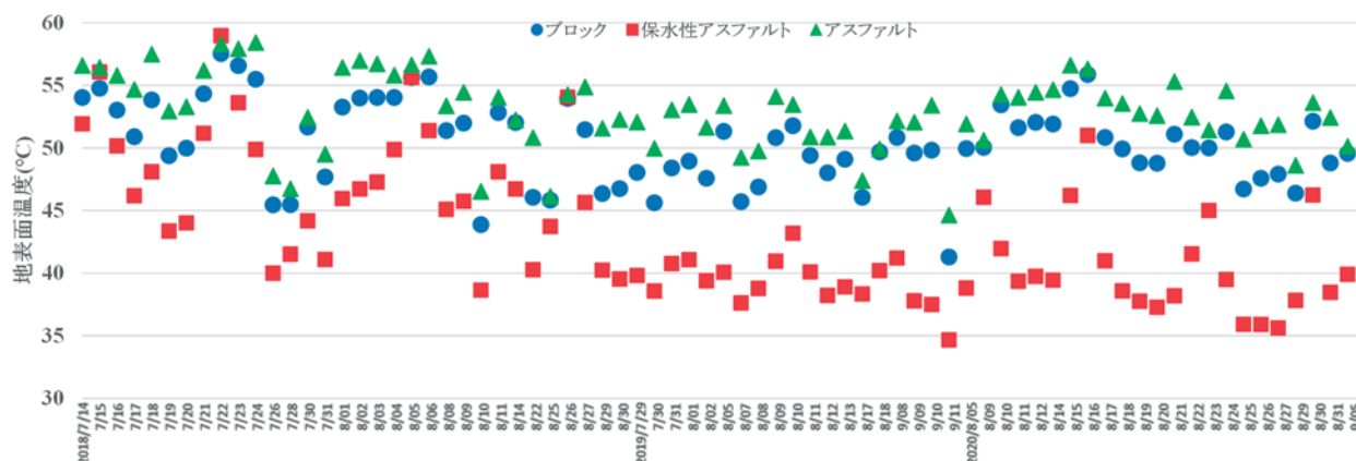
図5 日中における地表面温度平均値の推移
