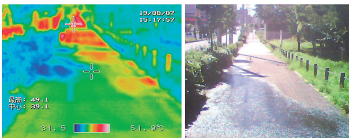
図4 保水性アスファルトにおけるサーモカメラ画像
