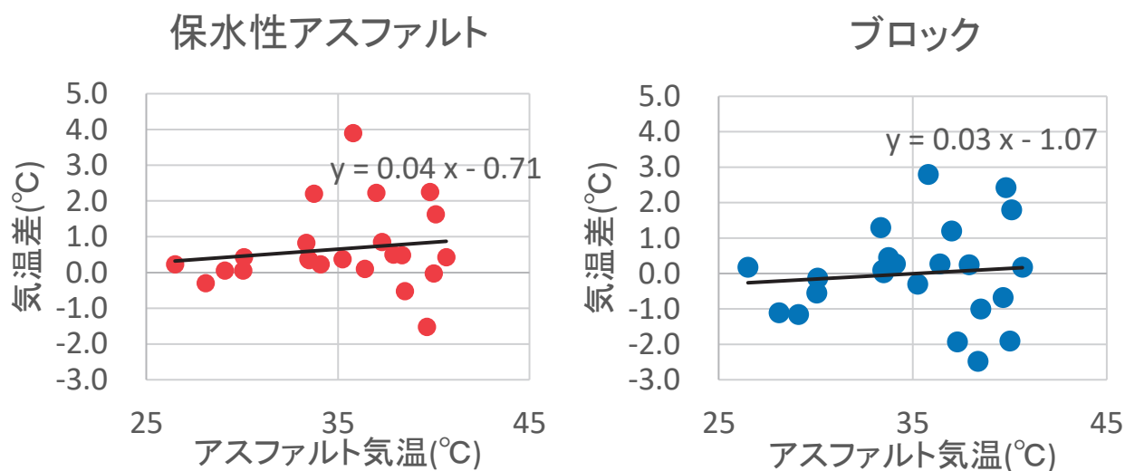
図7 アスファルトと保水性アスファルト又はブロックとの気温差(地上 1.1m)
