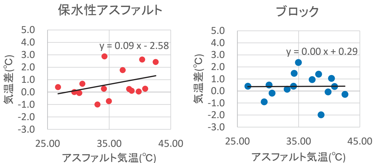
図6 アスファルトと保水性アスファルト又はブロックとの気温差(地上 0.6m)
