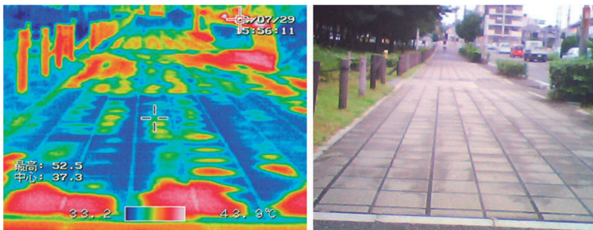
図3 ブロックにおけるサーモカメラ画像
