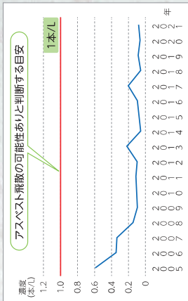
図4 アスベスト環境濃度(年平均値)の推移
