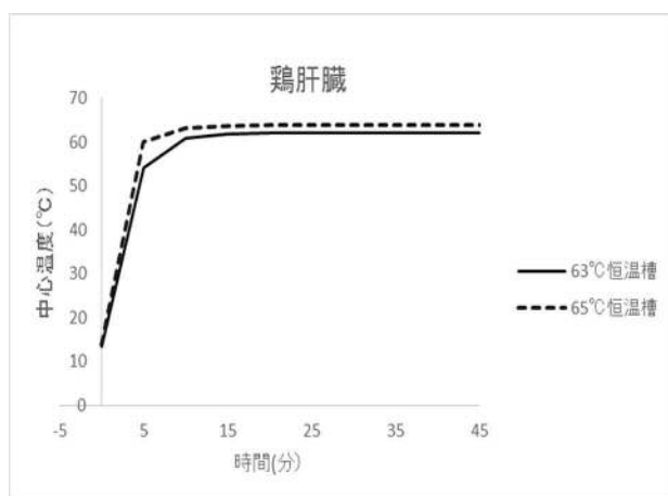
図3 鶏肝臓の中心温度変化
