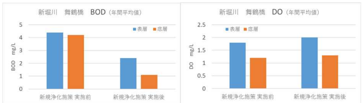
水質シミュレーションによる新堀川の上流部（舞鶴橋）における水質変化の傾向
