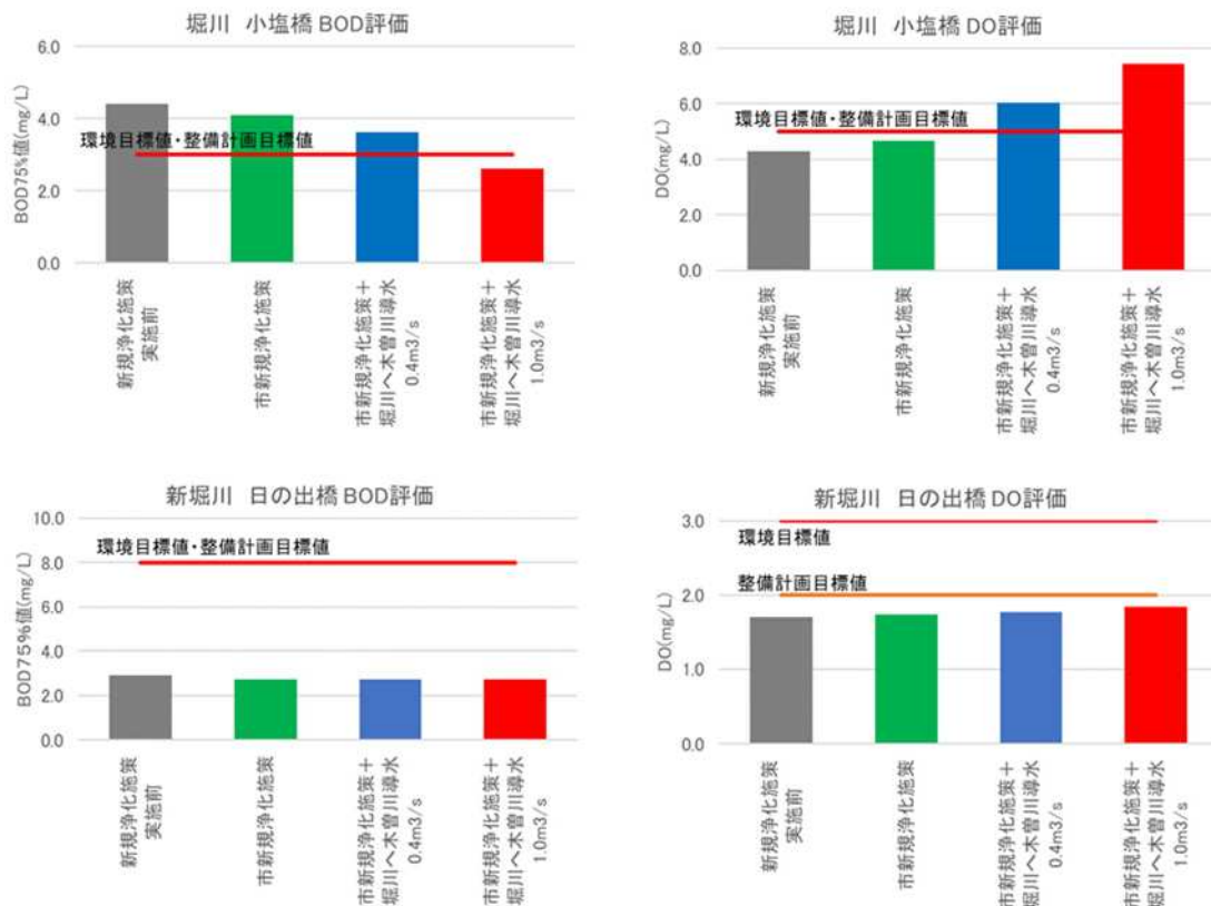
水質シミュレーションによる「小塩橋」「日の出橋」におけるBODとDOの水質予測結果
