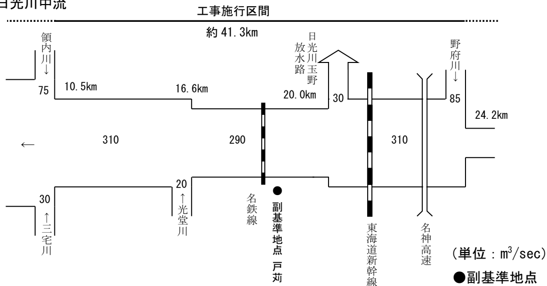
図-14 河川整備計画の目標とする流量配分図（日光川中流）
