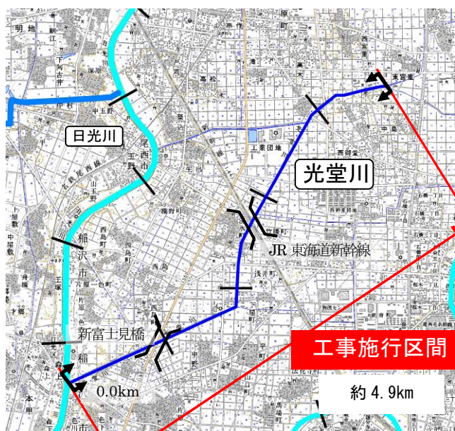
図-23 光堂川平面イメージ
