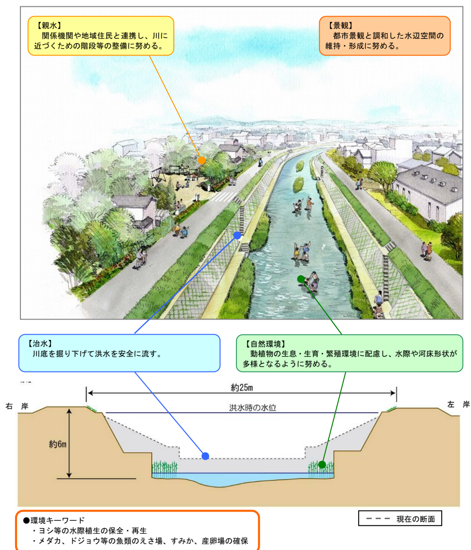
図-13 日光川上流イメージ(25.6km付近)
