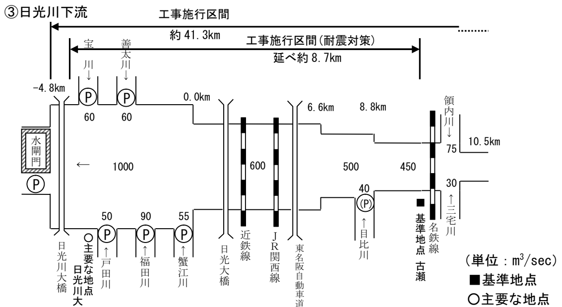
図-16 河川整備計画の目標とする流量配分図(日光川下流)
