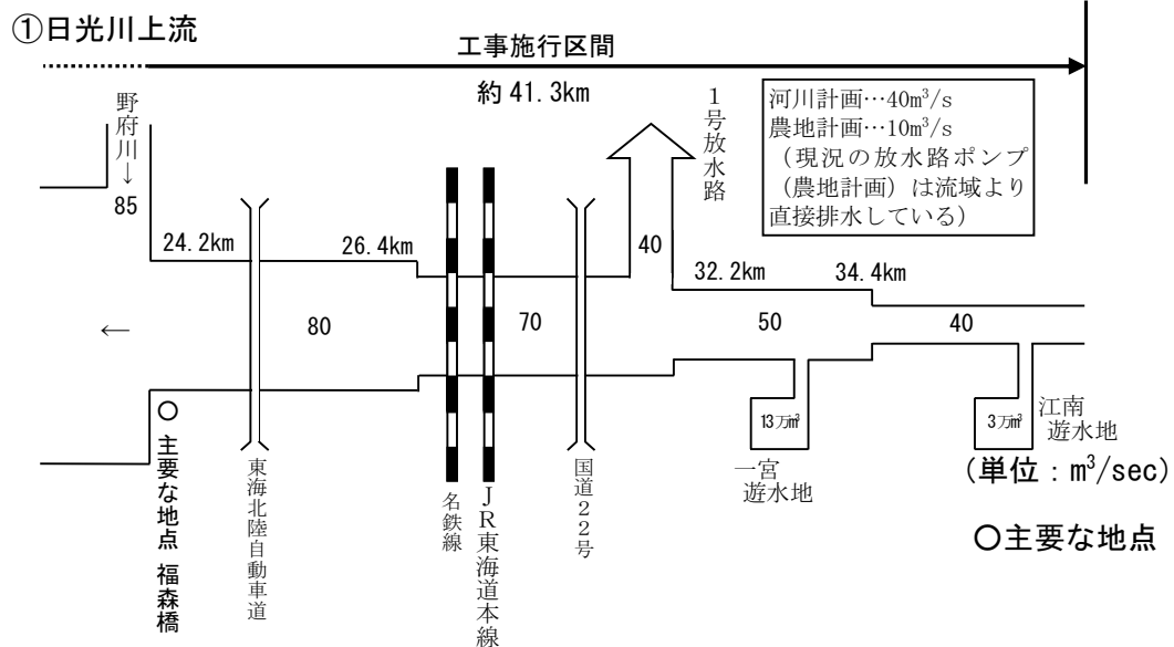
図-12 河川整備計画の目標とする流量配分図(日光川上流)
