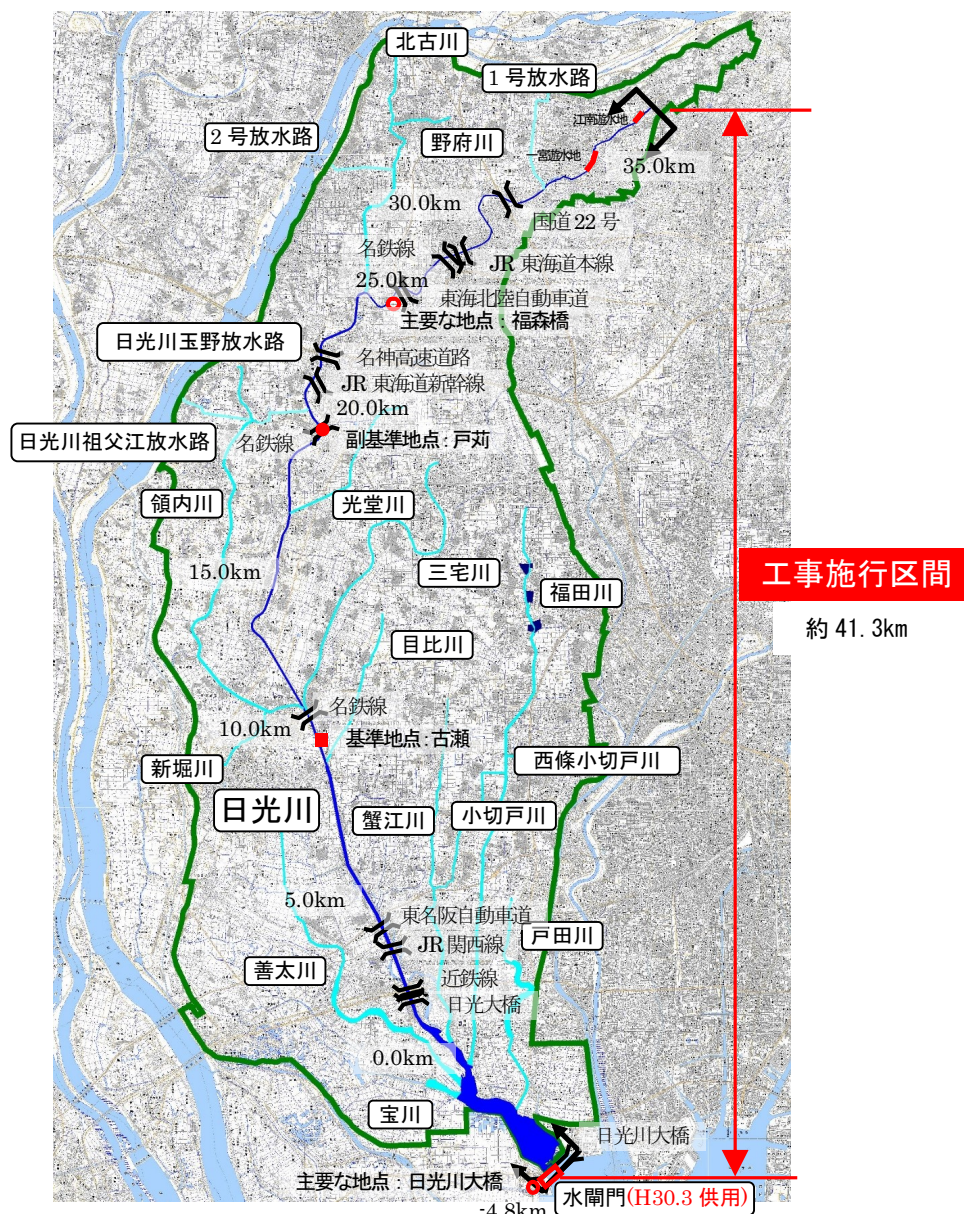
図-11 日光川本川平面イメージ
