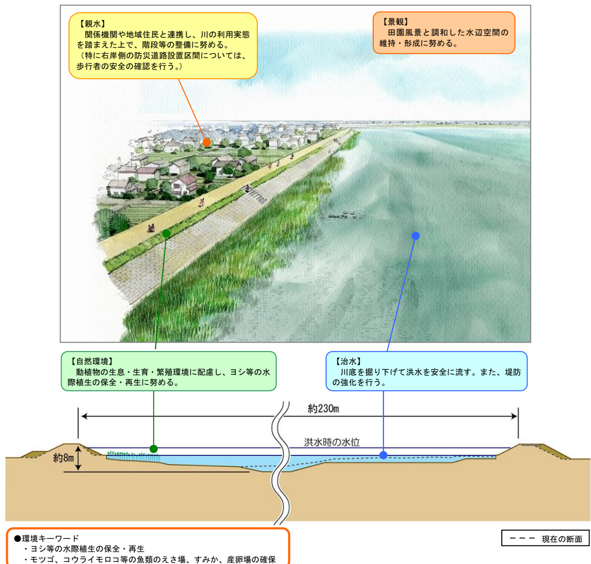
図-17 日光川下流イメージ(-1.0km付近)
