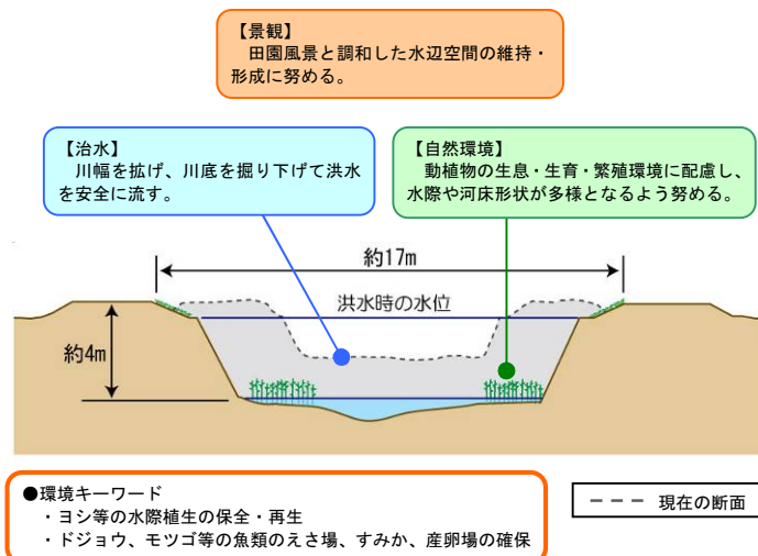
図-24 光堂川イメージ（4.0km 付近）
