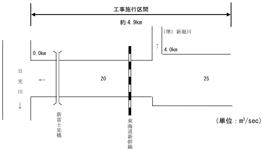
図-22 河川整備計画の目標とする流量配分図（光堂川）
