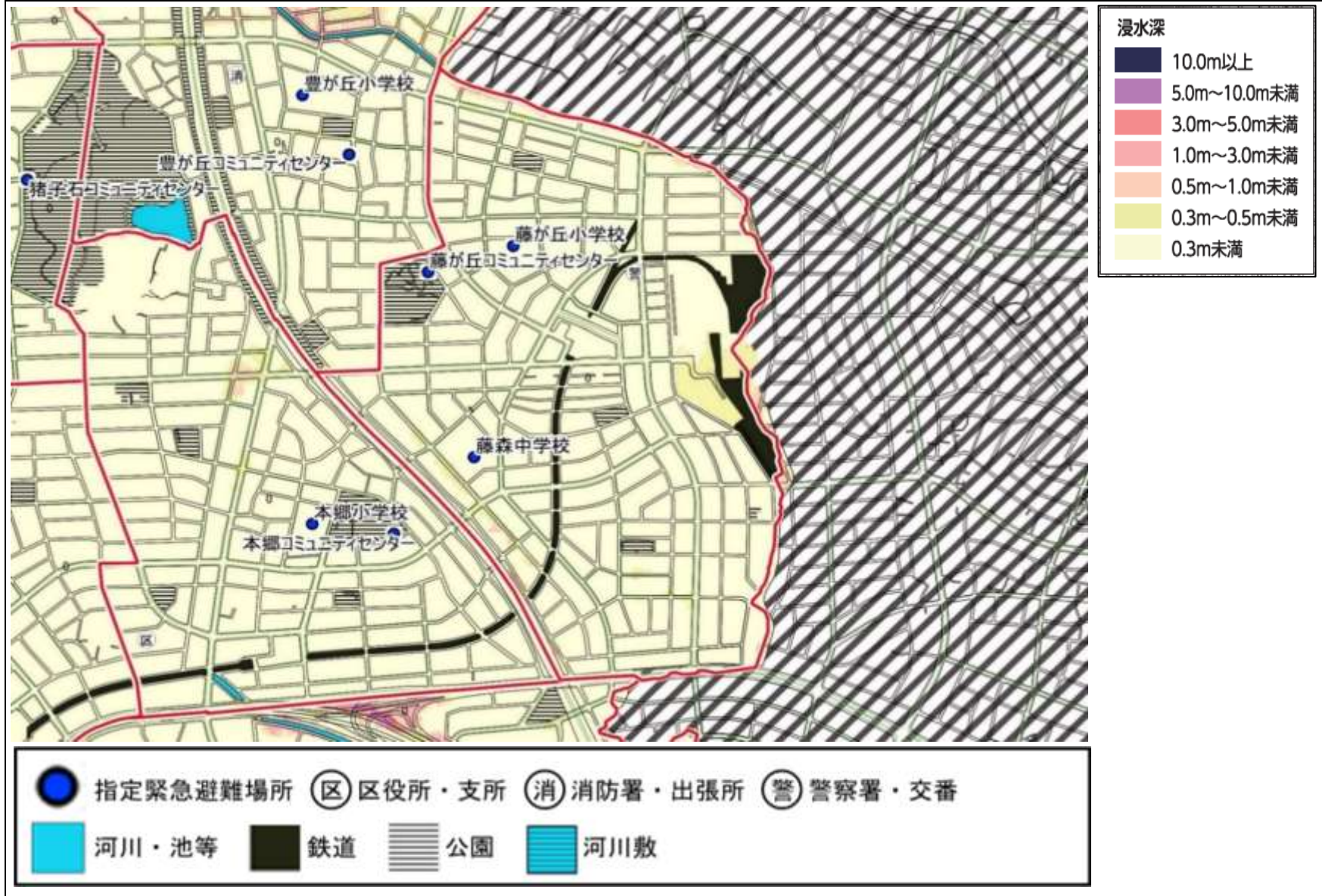
(4) 内水氾濫浸水想定（内水氾濫時に想定される浸水深）
