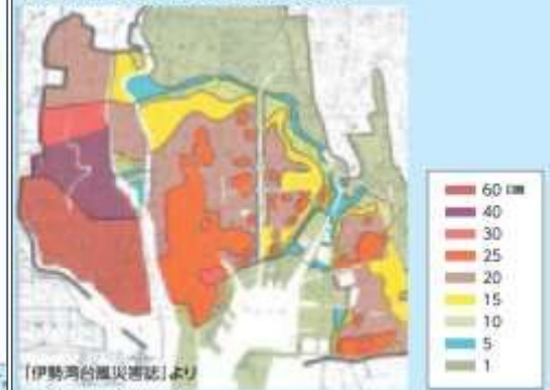
伊勢湾台風時の浸水日数
