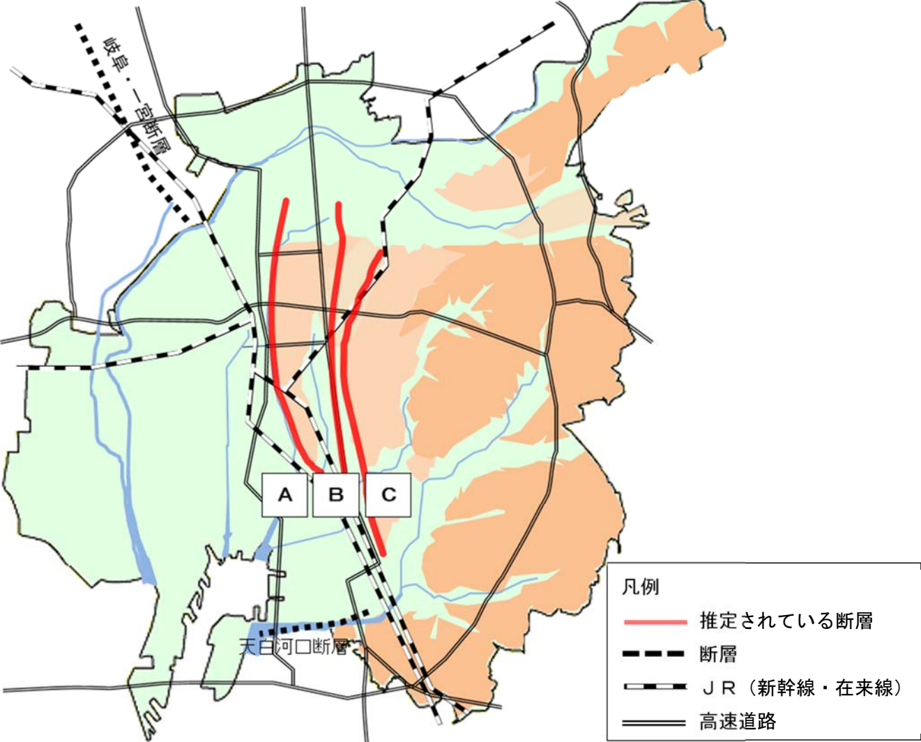
《名古屋市付近に推定されている断層の概略図》
