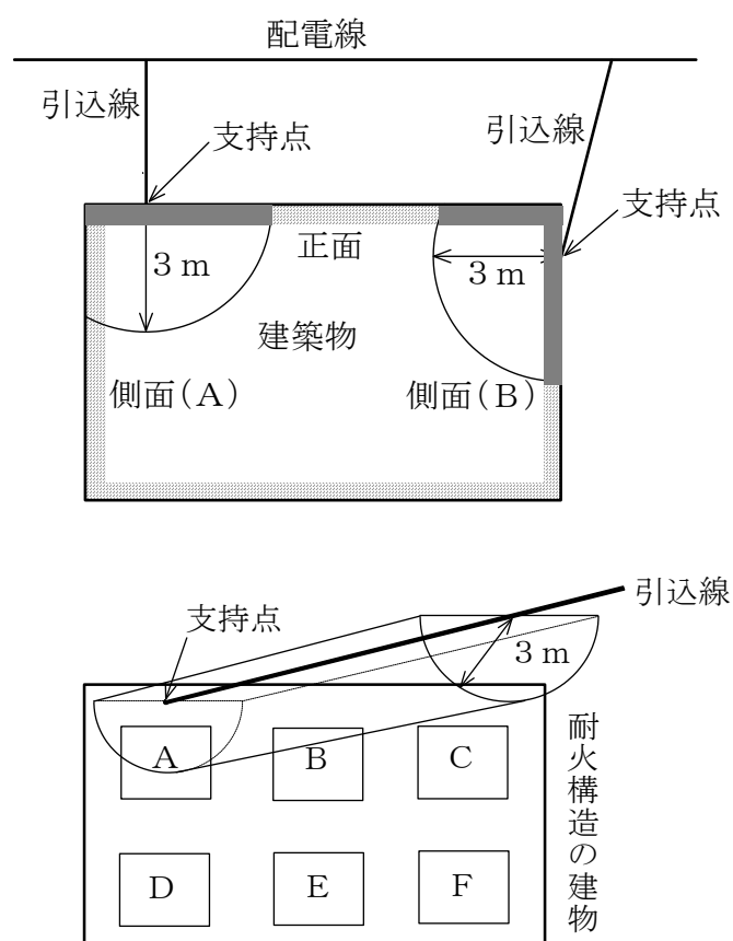
第23-4図 下部3 m以内の外壁規制の例
