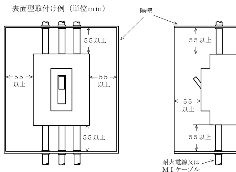
第23-2図b 配線用遮断器の取付け例
