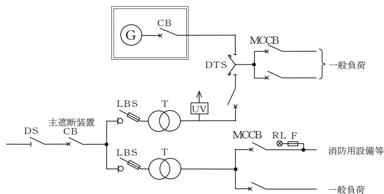
第23-7図c（高圧又は特別高圧で受電する場合）
