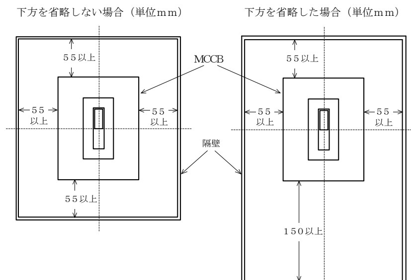
第23-2図b 配線用遮断器の取付け例
