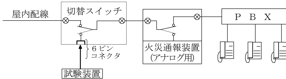
第13-7図 (火災通報装置 (アナログ用) と試験装置を接続する装置の設置方法)
