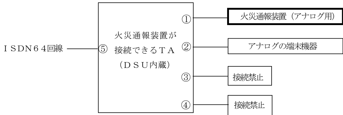
第13-5図b (TAにDSUが内蔵されている場合の各接続端子の接続例)
