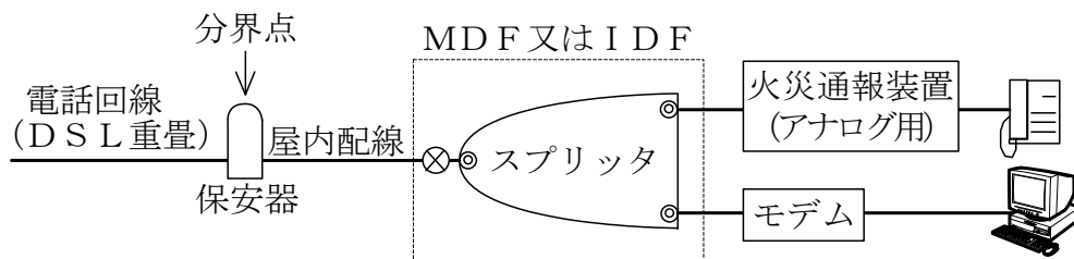
第13-3図 (スプリッタがある場合)
