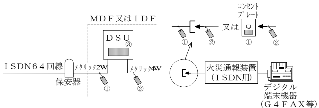
第13-9図d I S D N 6 4 回線に火災通報装置（I S D N 用）を接続する場合
