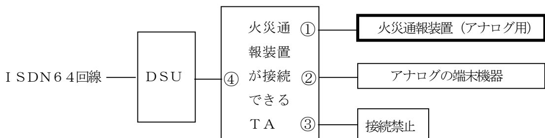
第13-5図c (TAにDSUが内蔵されていない場合又はTAに組込まれたDSUを使用せず、別に設置したDSUを使用する場合の各接続端子の接続例)
