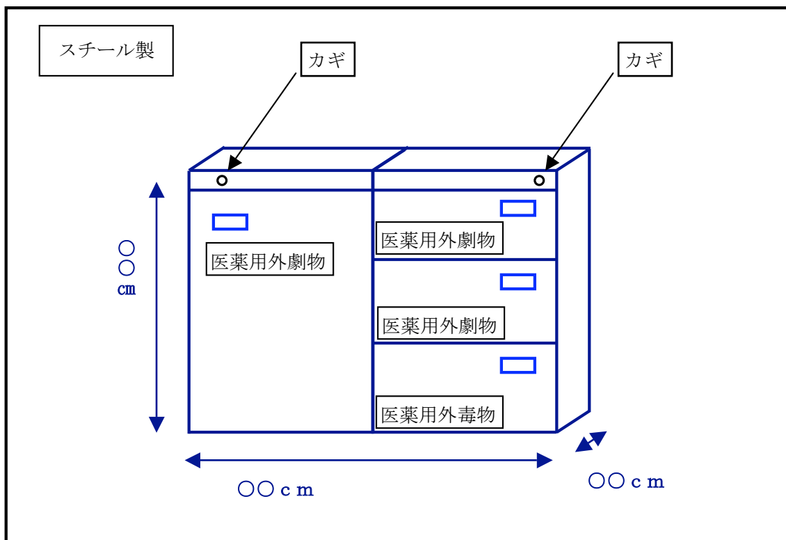
貯蔵陳列設備の立面図
