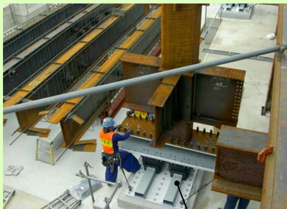
写真鉄骨工事状況
