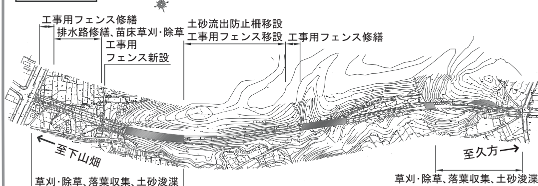
土砂流出防止柵の移設
