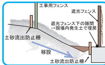
土砂流出防止柵の移設
