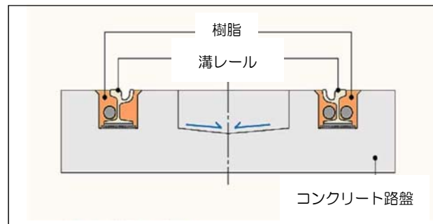
樹脂固定軌道
