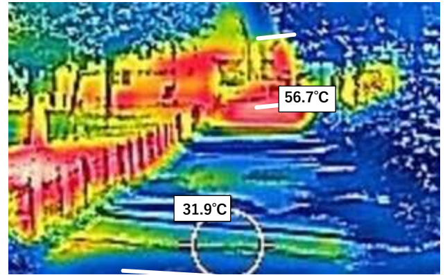
保水性アスファルト舗装（A）の写真（左）とサーモカメラ画像（右） 撮影日：9月18日（送水時間：54min/h）
