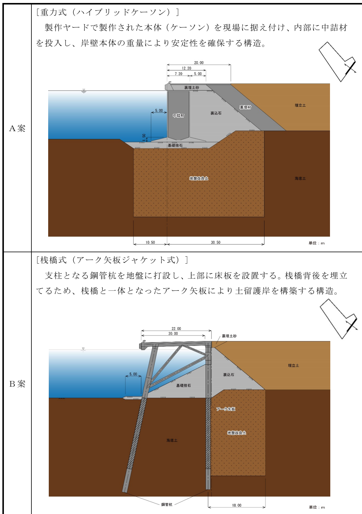
図 1-2-7 標準断面図
