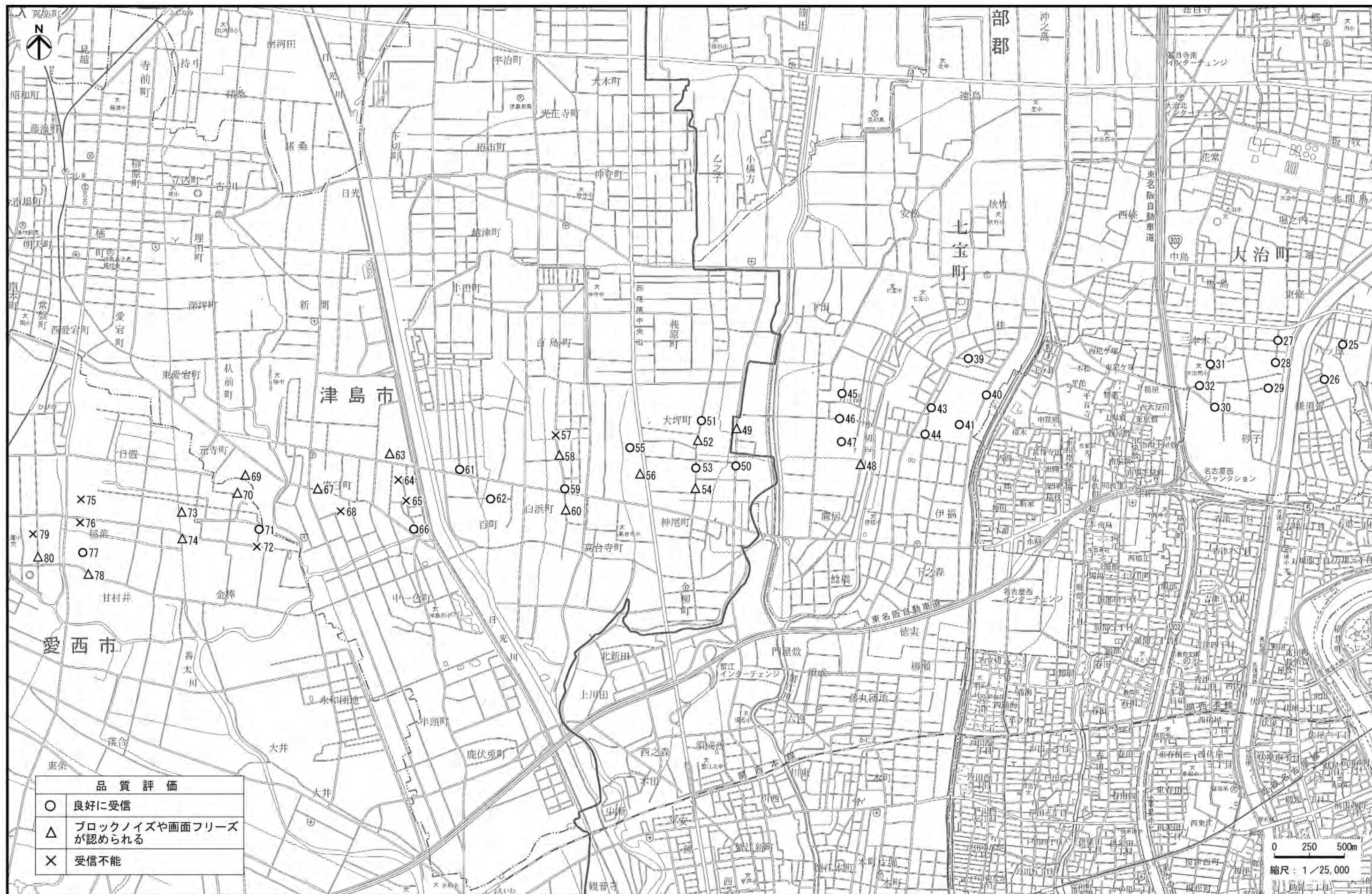
図－１（２） 名駅局における地上デジタル放送電波の受信品質評価（名古屋市内外）
