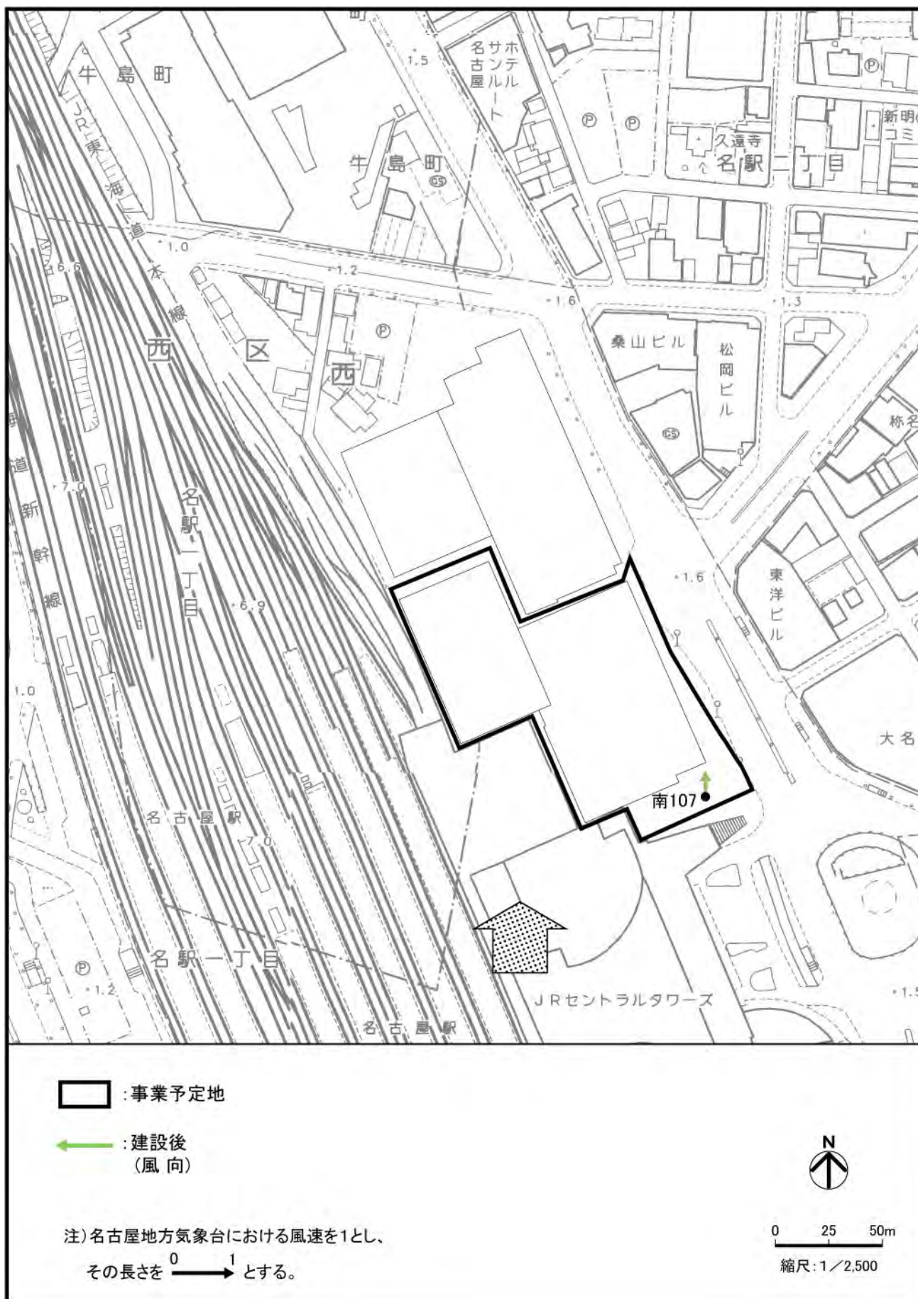
図-2(2) 空地内の風向及び風速 (S) (新建築物建設後)
