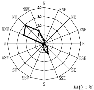
風力階級 4 以上による年間風配図（地上60m）
