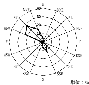
風力階級4以上による年間風配図（地上80m）
