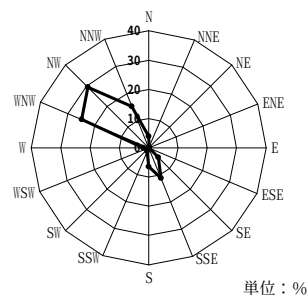
風力階級4以上による年間風配図（地上50m）
