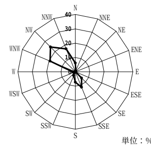
風力階級4以上による年間風配図（地上90m）
