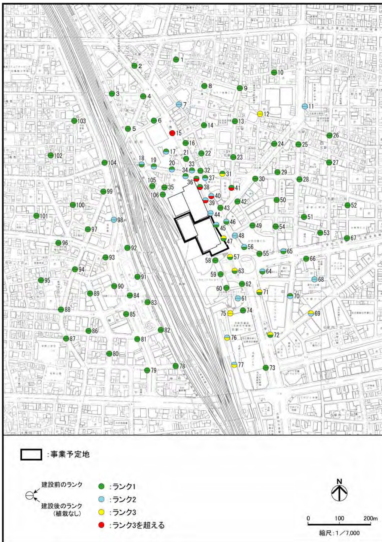
図ー1 風環境のランクの変化（新建築物建設前・建設後（植栽なし））
