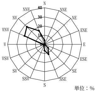
風力階級 4 以上による年間風配図（地上70m）
