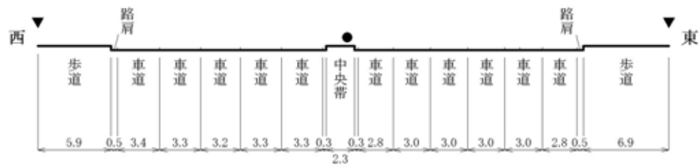
No.10断面
