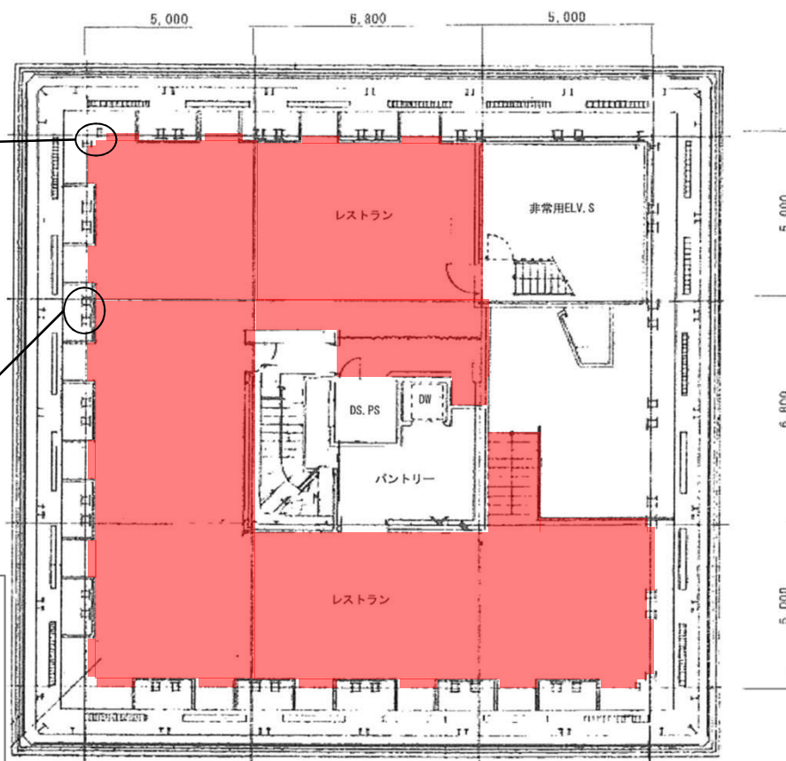
東山スカイタワー7階平面図
