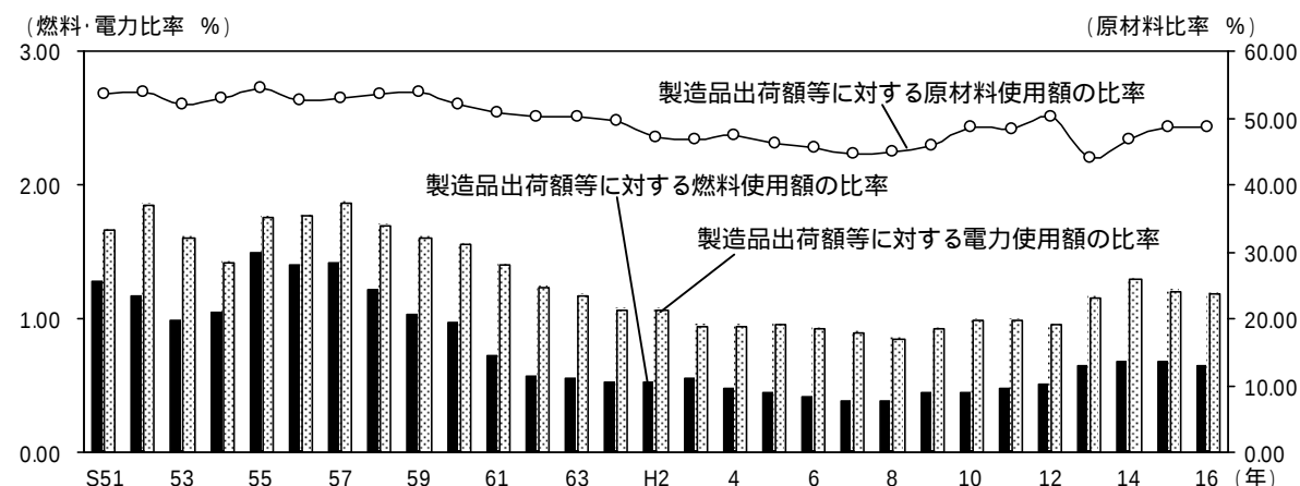
図8 製造品出荷額等に対する原材料・燃料・電力使用額の比率の推移(従業員30人以上の事業所)
