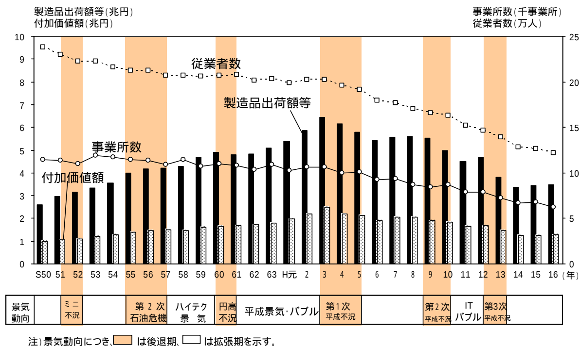
付表2 全国、愛知県、名古屋市の従業者規模別主要4指標の比較(従業者4人以上の事業所)
