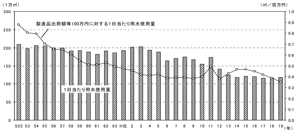
図 10 1 日当たり用水使用量の推移 (従業員 30 人以上の事業所)
