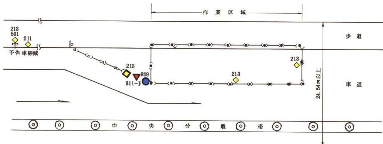
大型道路標識の事例
