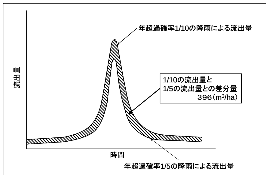
図 2.2 年超過確率 1/10 の降雨と年超過確率 1/5 の降雨の流出量の関係
