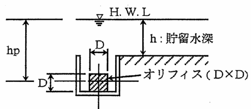
貯留施設の場合
