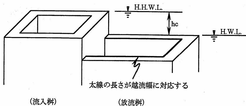
図 6.6 流出抑制柵
