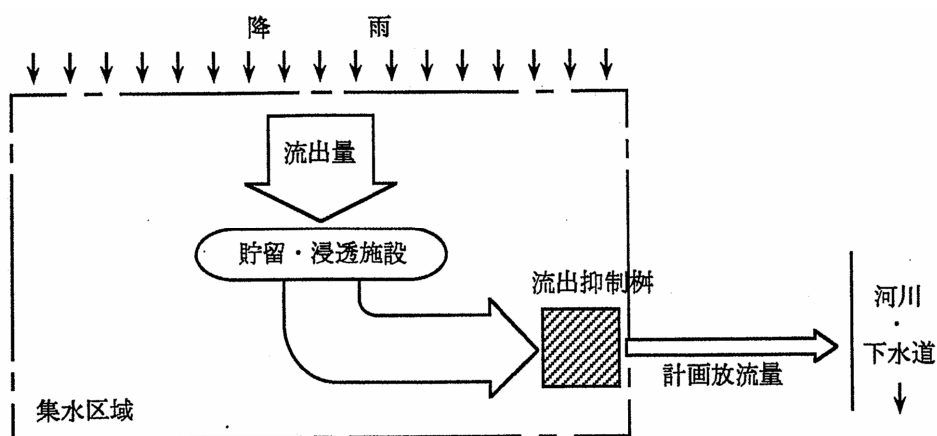
図 1.2 流出抑制柵の機能
