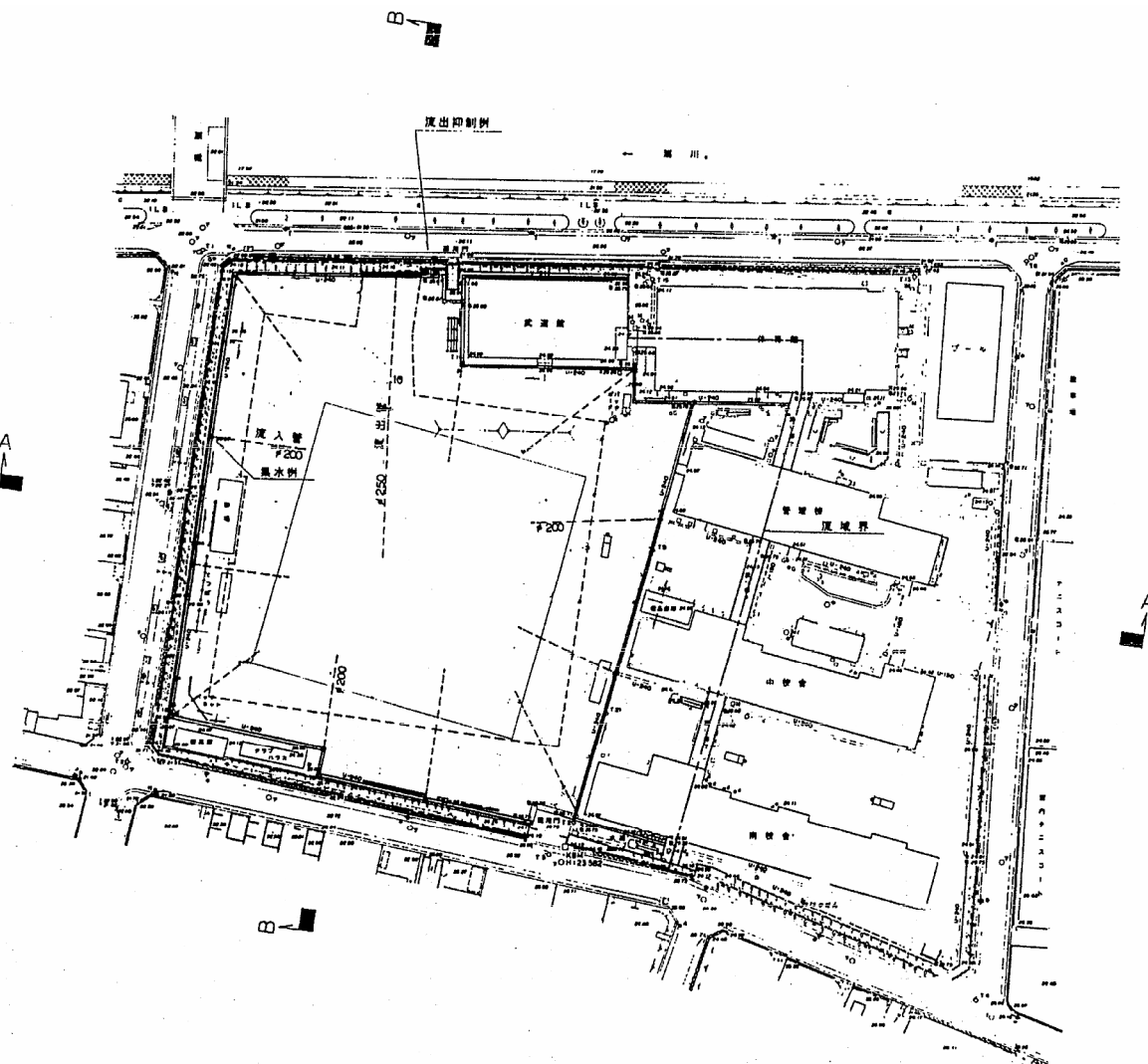
図8.3 扇台中学校 貯留施設平面図
