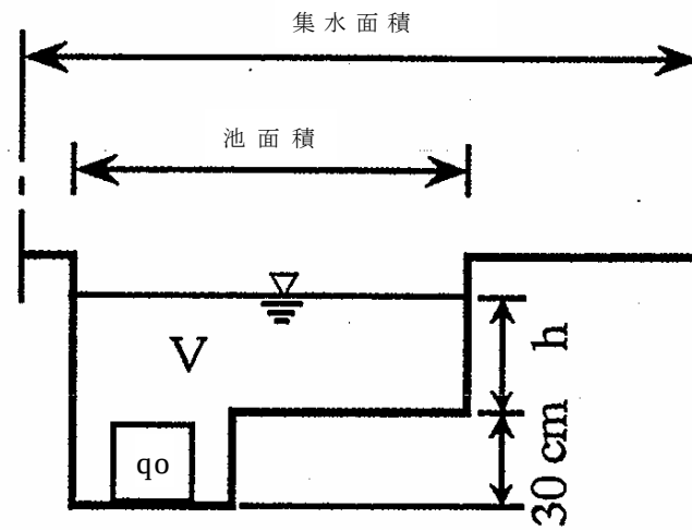
図 2.4 放流施設の概念図
