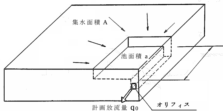
図 2.3 貯留施設の概念図
