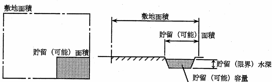
図 2.9 貯留可能容量
