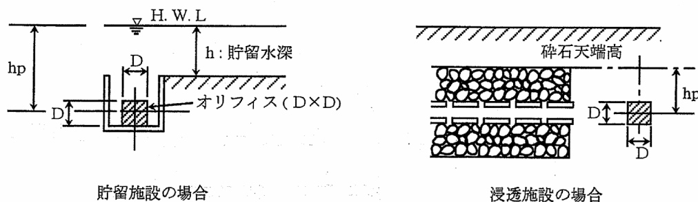
図 6.4 圧力水頭の決め方
