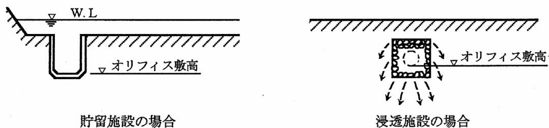
図 2.11 オリフィス敷高
