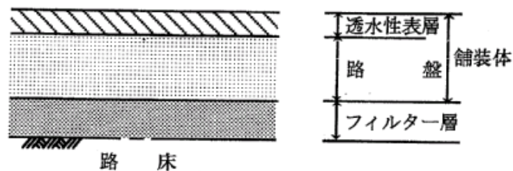
図 3.9 透水性舗装の概念
