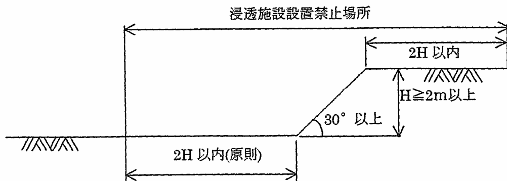
図 2.13 斜面近傍の浸透施設設置禁止場所の目安
