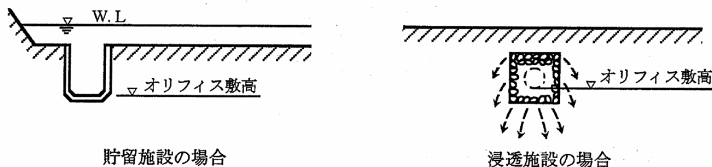
図 6.3 オリフィス敷高
