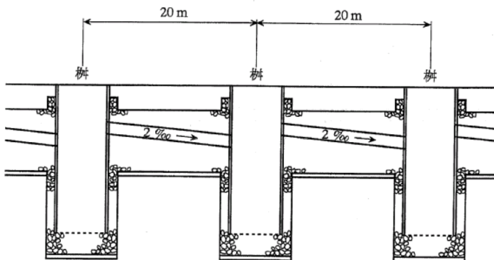
図 3.8 浸透トレンチの接続
