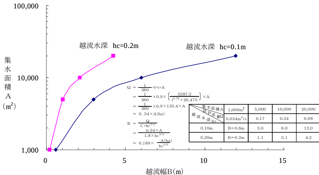
図 6.2 越流幅と集水面積の関係
