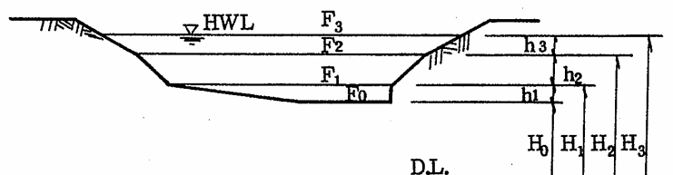
図 6.1 貯留施設断面図
