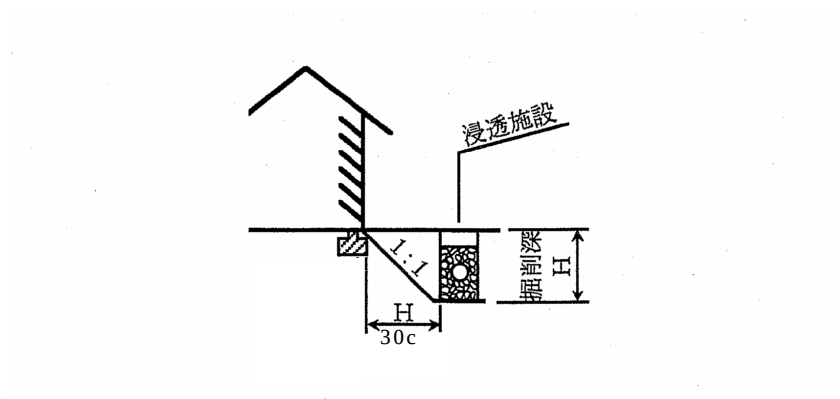
図 2.14 道路浸透柵および浸透トレンチの設置場所
