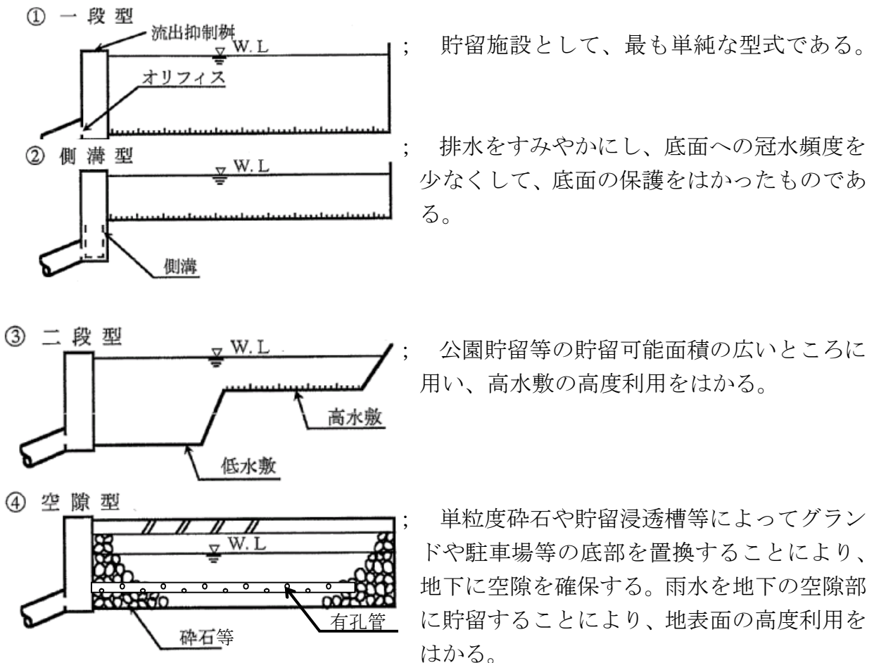
図 3.1 貯留施設の構造型式による分類
