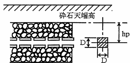
浸透施設の場合
