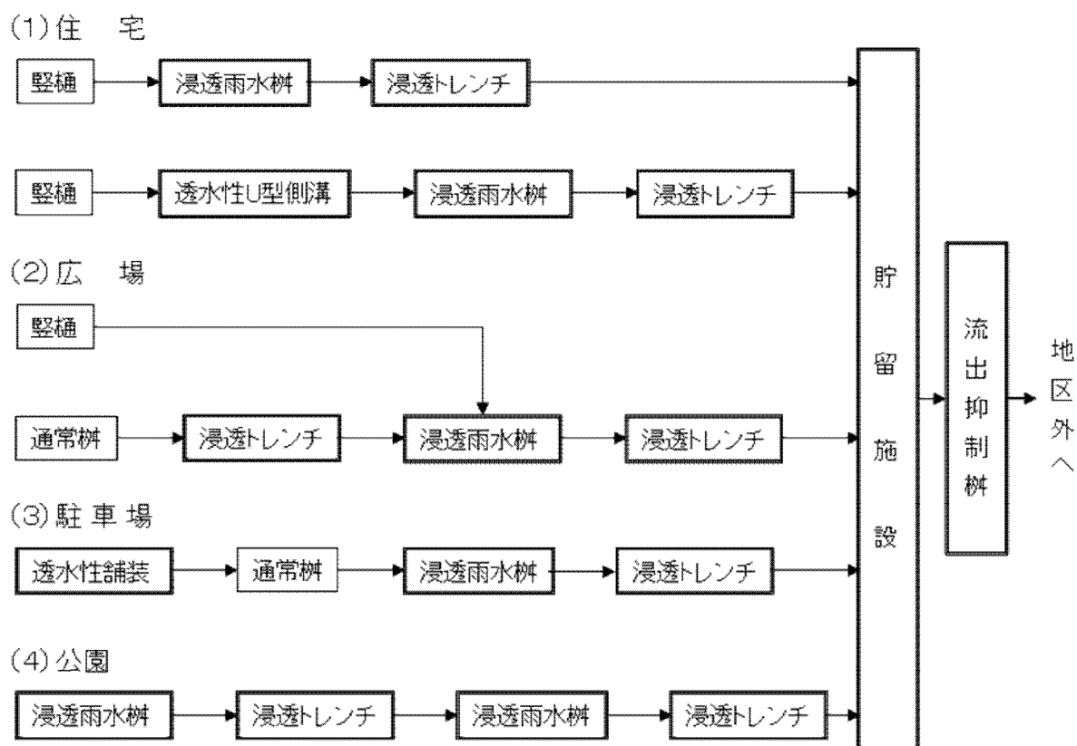
図 2.8 貯留浸透施設の組み合わせ例
