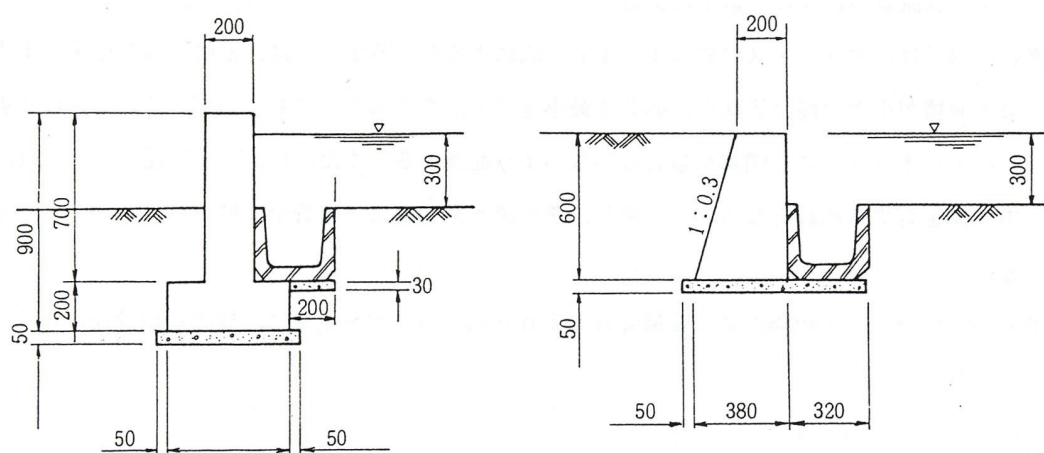
図 3.3 周囲小堤としてのコンクリート壁、コンクリートブロックの例
