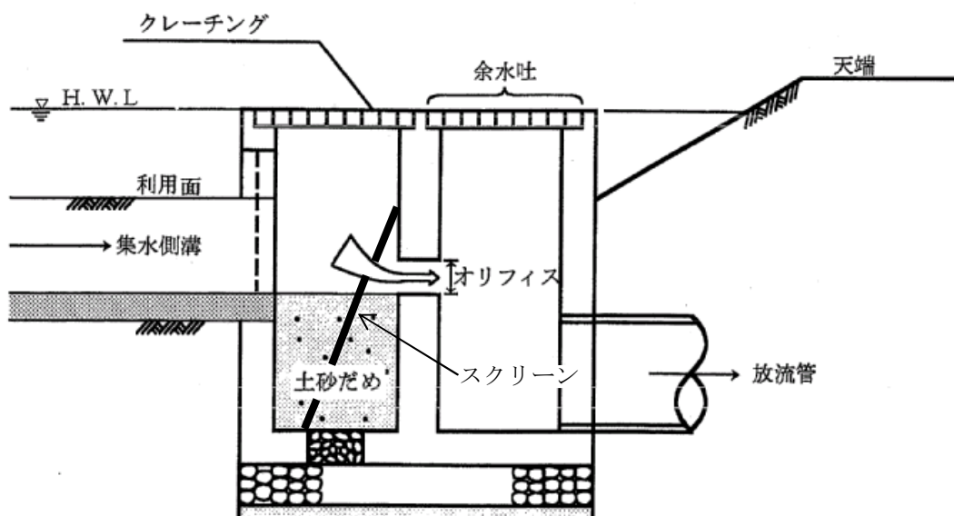
図 3.10 流出抑制柵
