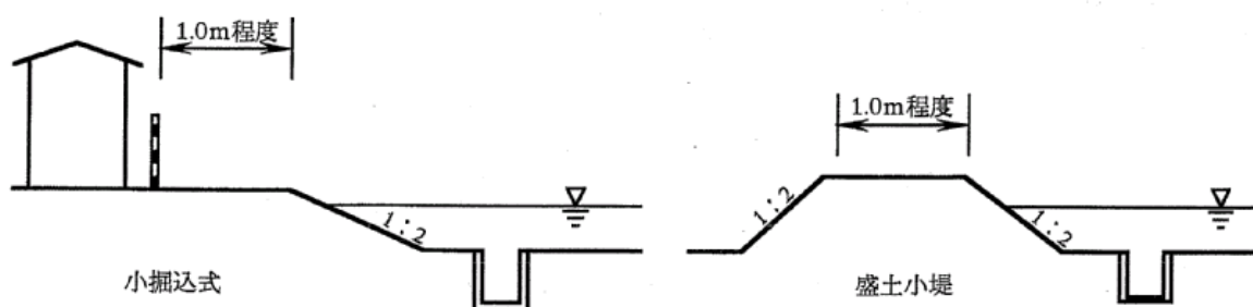
図 3.2 貯留部周囲小堤の概念
