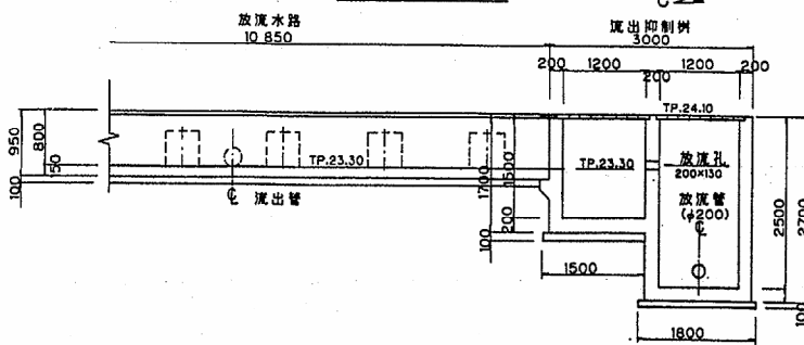
図 8.4 扇台中学校 貯留施設構造図
