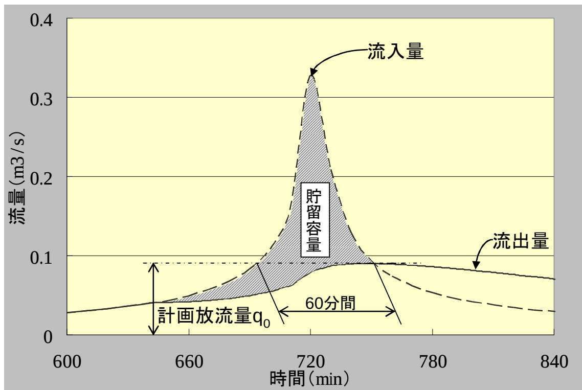
図 2.5 貯留容量と放流量の関係
