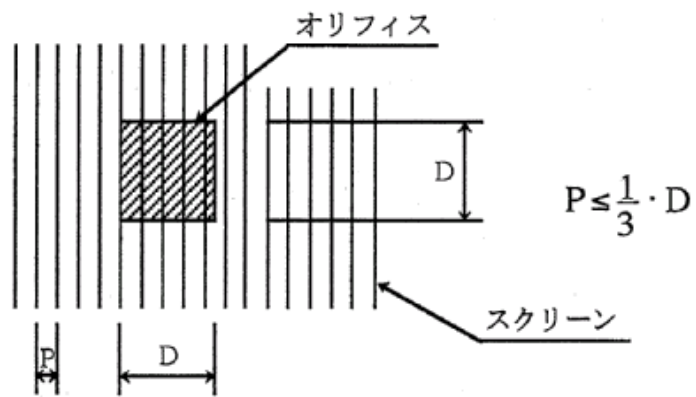
図 3.11 スクリーン間隔
