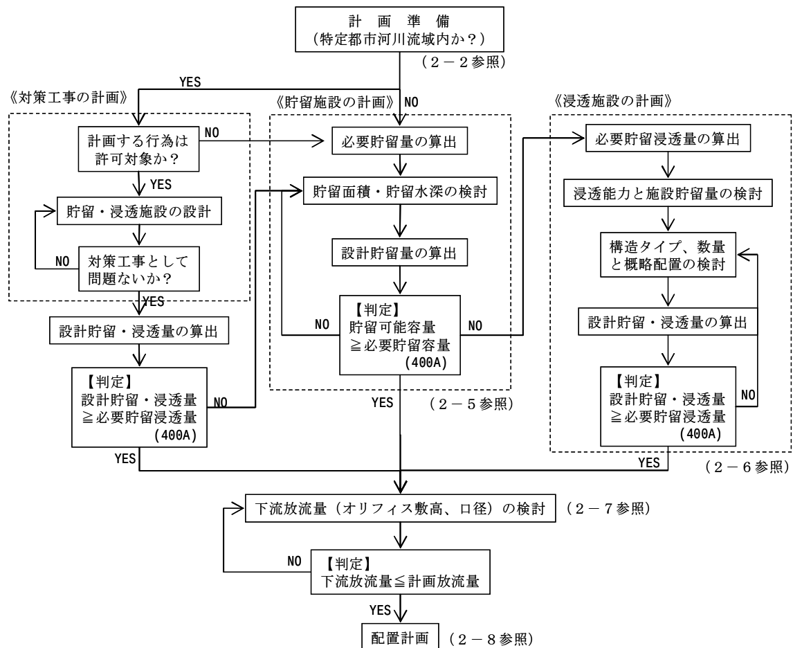
図 2.1 計画の概略手順
