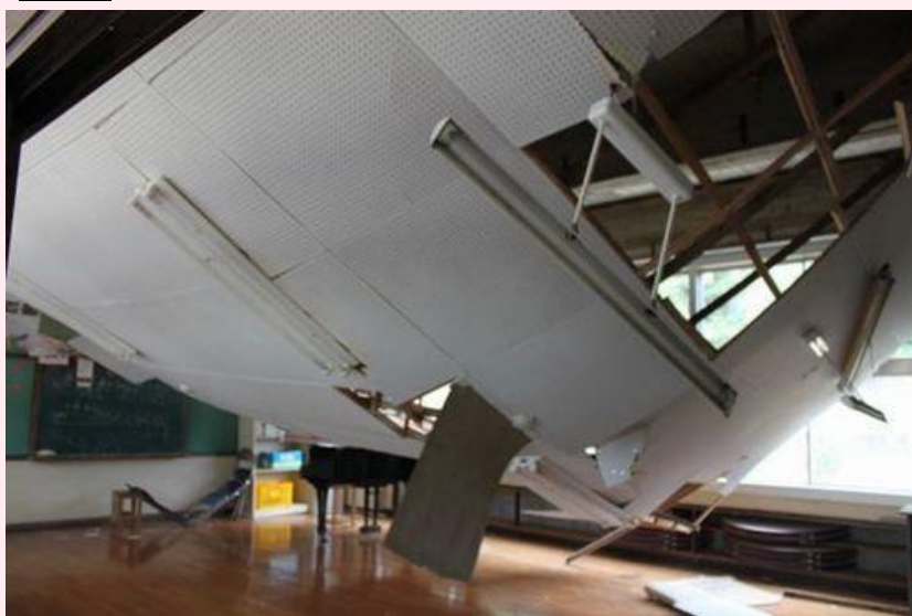
雨漏りにより天井の木製吊り部材が腐食して落下(築50年) この事例の原因は、地震ではなく、雨漏りです。 屋上防水層が劣化すると、校舎内で雨漏りが発生します。 雨漏りは水たまりを発生させ転倒の原因になるほか、劣化部材の落下、天井・床の汚損など様々な二次被害により学校運営の支障になります。
