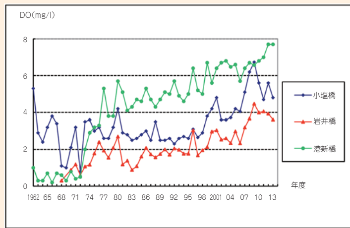
堀川のDO(溶存酸素量)の経年変化
