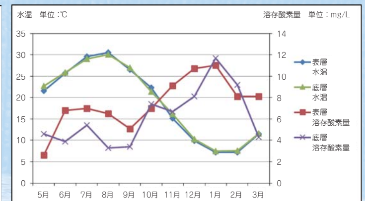
平成25年度の水温・溶存酸素量の表層と底層の比較
