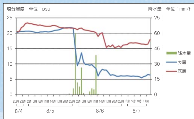
降雨による塩分濃度の変動(平成25年8月4日から8月7日)
