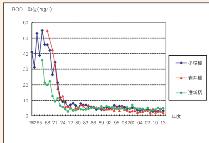
堀川のBOD経年変化
